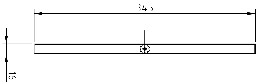
aanzicht binnenrooster
