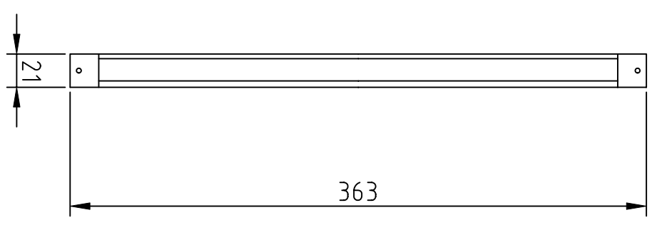
aanzicht buitenrooster
